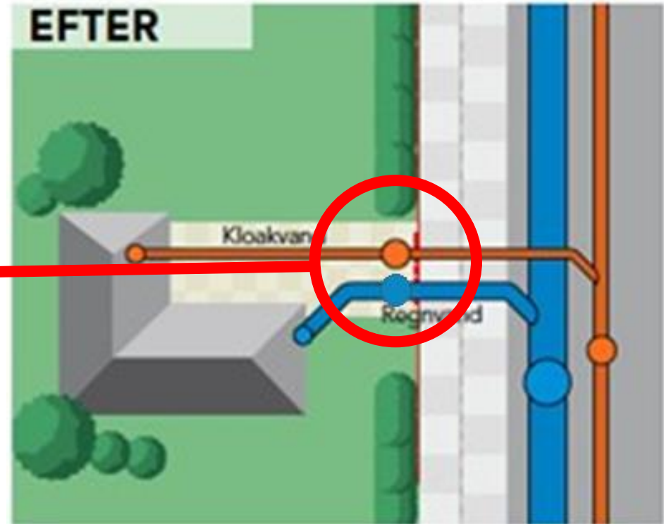
Separatkloakeret
