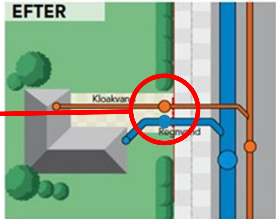
Separatkloakeret
